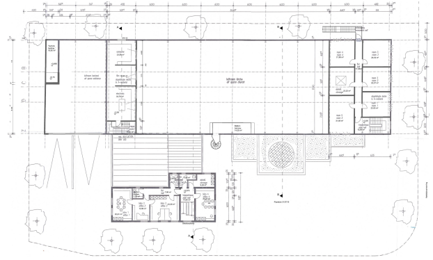
Obergeschoss
